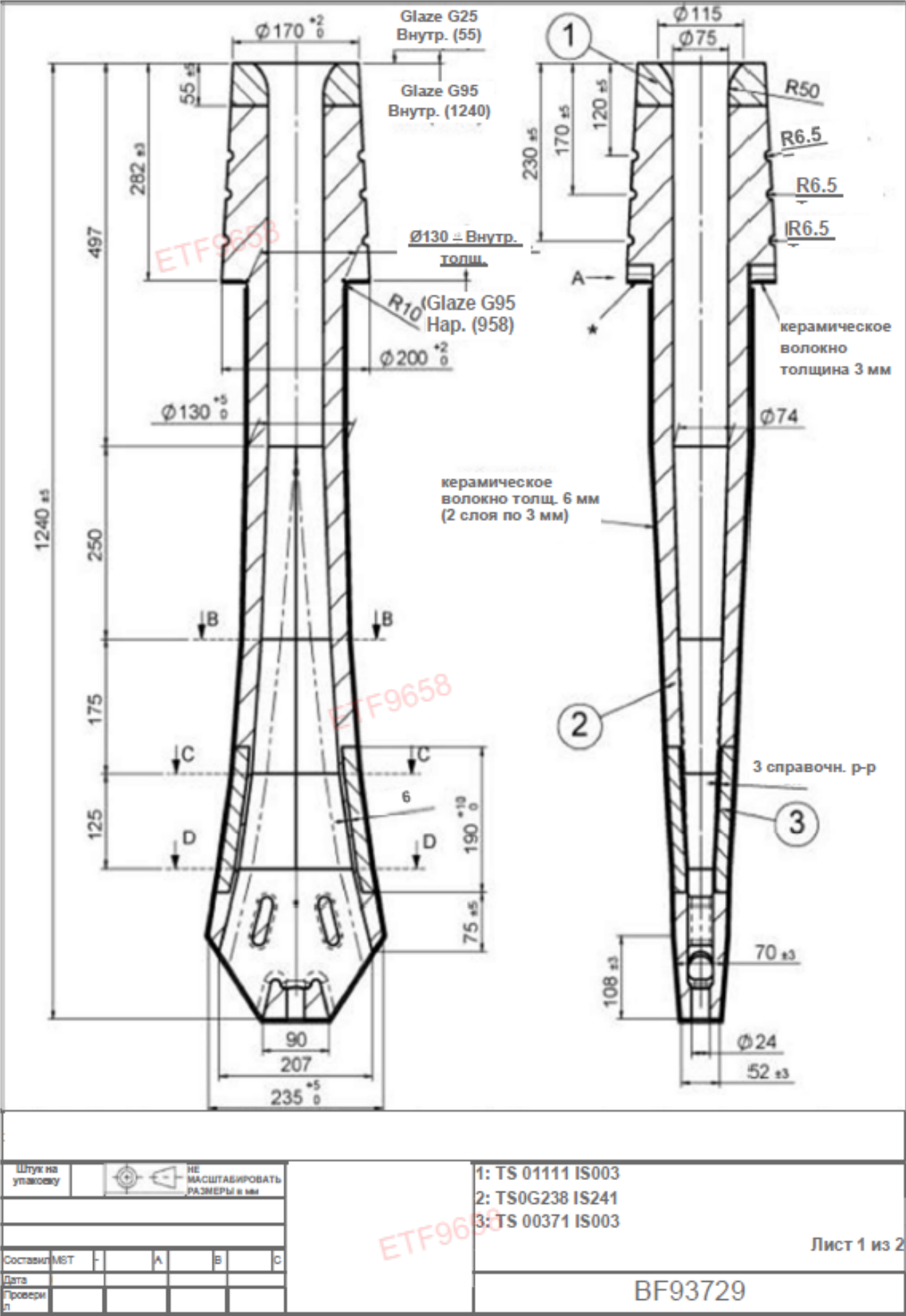
Приложение №1 Чертеж огнеупорного погружного стакана SEN Скандинавский тип головки.
